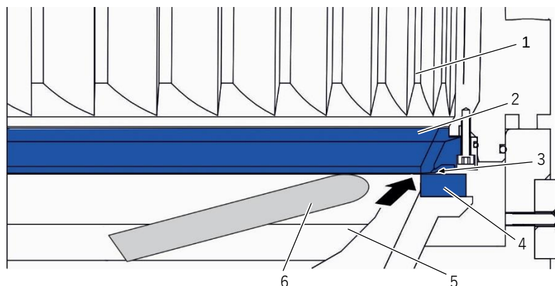
Рис. 12 Установка размера зазора с помощью измерительного щупа
