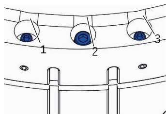
Рис.11. Ослабление регулировочных и стопорных винтов
